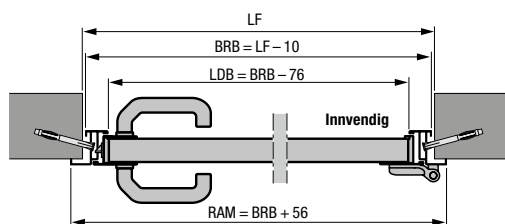
Sidedør med hjørnekarm av aluminium, profiltipe 1 eller 2 Innvendig montasje
