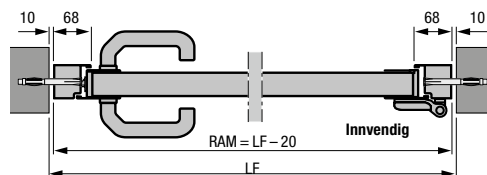
Sidedør med blokkarm av aluminium, profiltipe 2 Montering i åpningen
