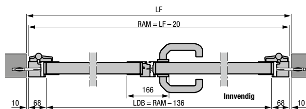
2-fløyet sidedør med blokkarm av aluminium, profiltipe 2 Montering i åpningen
