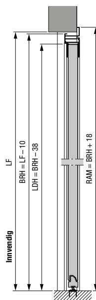
Sidedør med hjørnekarm i aluminium, profiltipe 2 Utvendig montering
