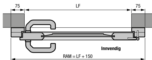
Sidedør i massivt tre Montering bak åpningen
