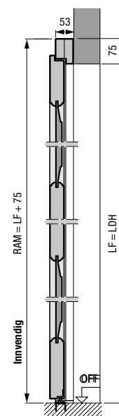
Sidedør i massivt tre Montering bak åpningen
